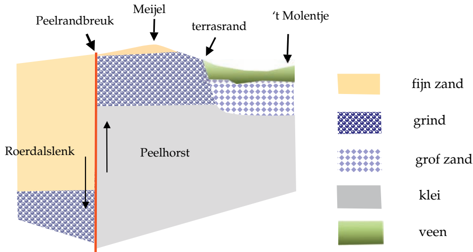
Figuur 3: Doorsnede peelslenk-peelhorst.
